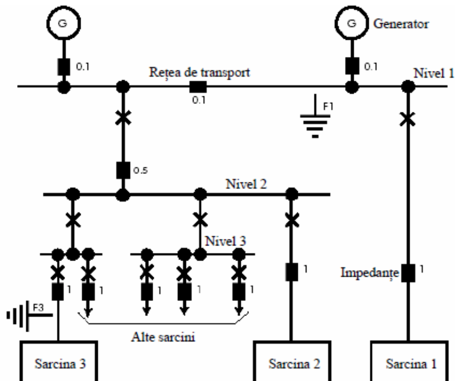
Fig.2. Cauze ale golurilor de tensiune
