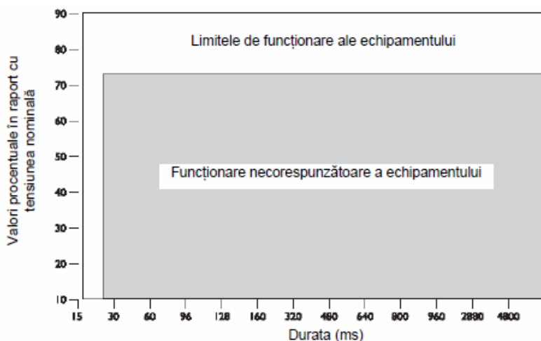
Fig.5 - Curbă de toleranță la goluri pentru unități PLC sensibile
