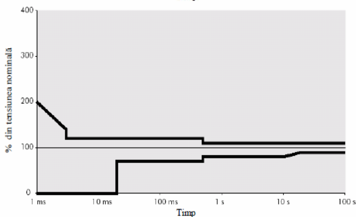
Fig.4. Curba ITIC
