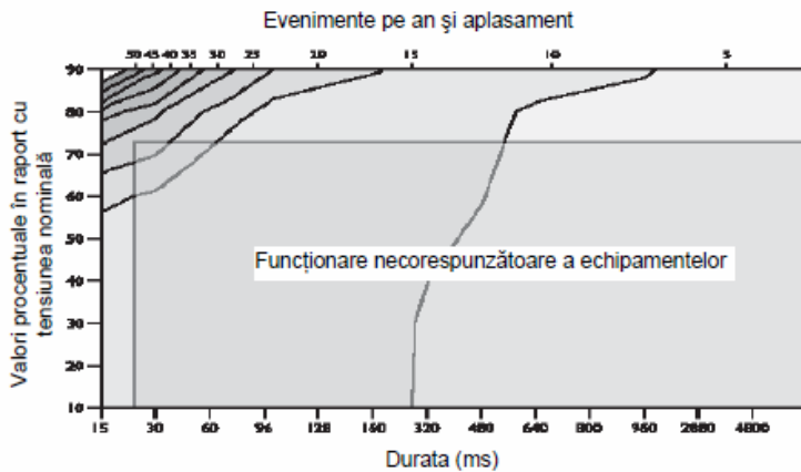
Fig. 6 – Curba de toleranță la goluri stabilită de graficul de contur al golurilor de tensiune
